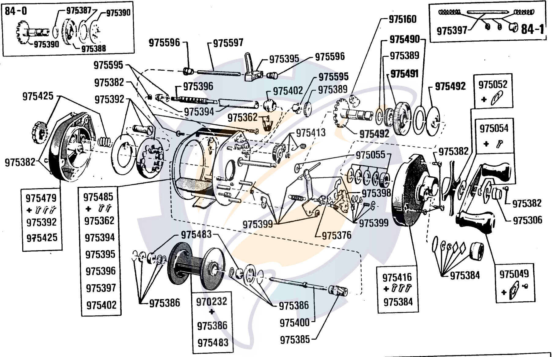
Ambassadeur MAG I PLUS 84-2
